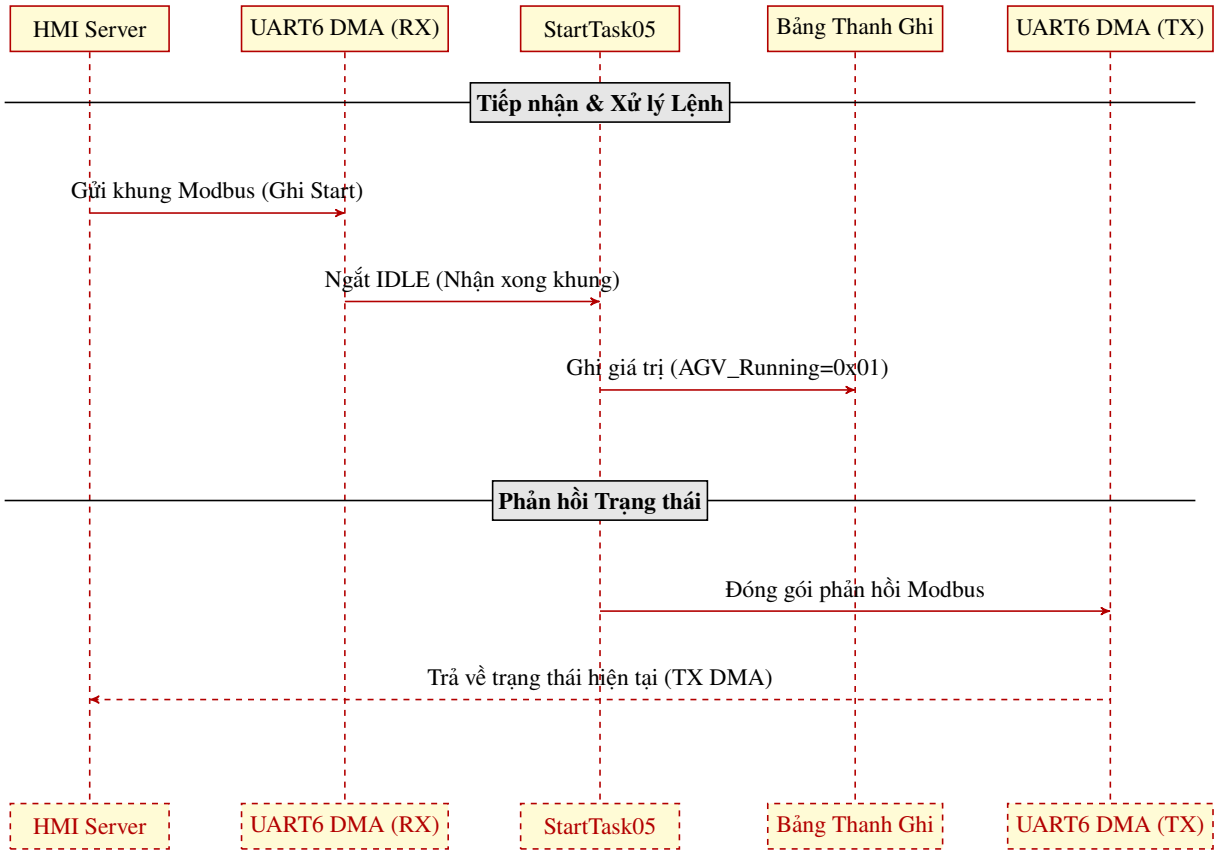
Hình 4.12 Sơ đồ tuần tự giao thức truyền thông Modbus RTU.
