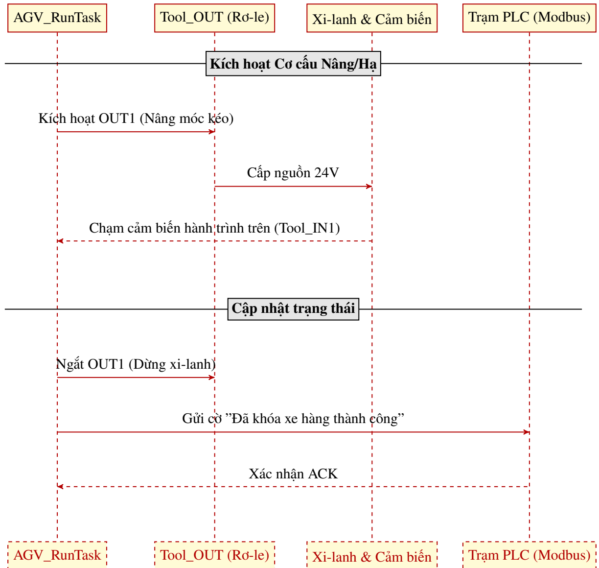
Hình 4.10 Sơ đồ tuần tự hoạt động của cơ cấu móc kéo xe hàng.
