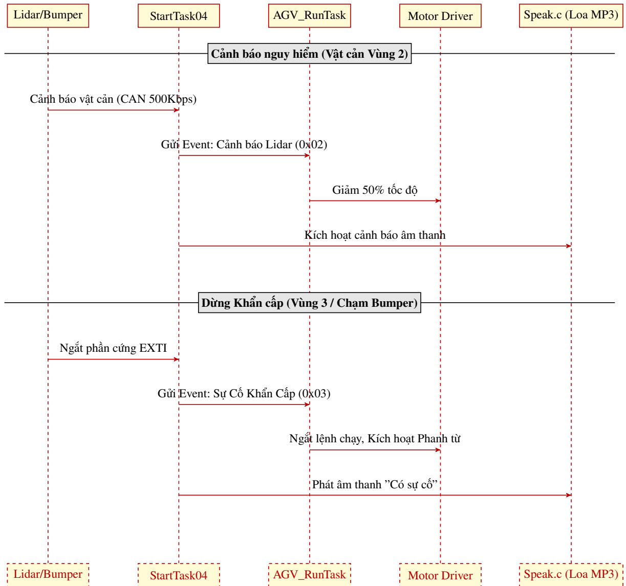
Hình 4.9 Sơ đồ tuần tự luồng giám sát an toàn và xử lý sự cố khẩn cấp.
