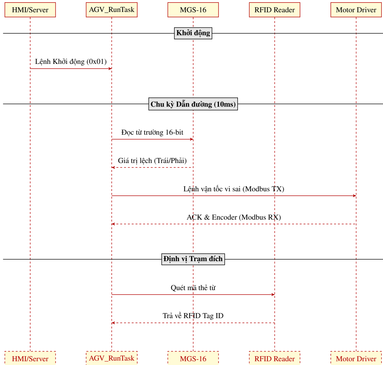
Hình 4.8 Sơ đồ tuần tự quá trình dẫn đường và nhận dạng trạm RFID.
